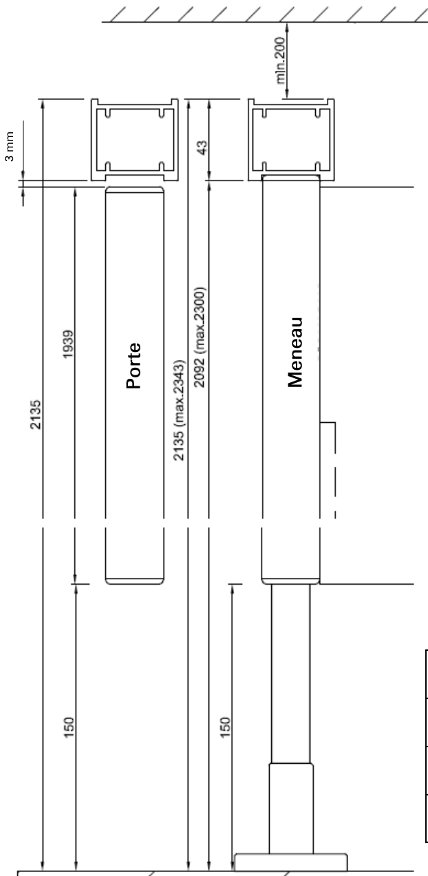
Coupe configuration standard
