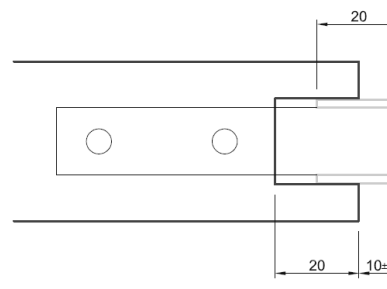
Profilé en joint-croix (option)
