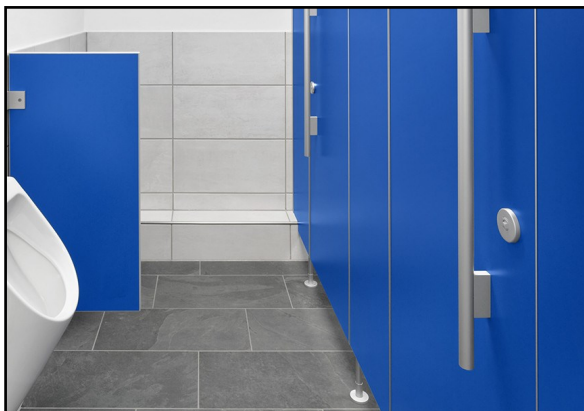
Effet flottant avec piètements, stabilisateur en retrait et barres GS 40 – 430 mm
