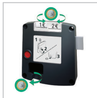
Ticket- / Pfand- und Kassierschloss
