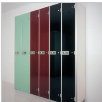
Nummernschild aus Aluminium mit Gravur, versenkte Spezialschraube und glattflächige Bandabdeckung
